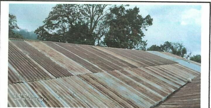
CUBIERTO DE LAMINAS: Sustitución de lámina existente por lámina troquelada. -Cambio de techado con lámina troquelada de 2 aulas con medidas 18 mts de largo por 5.80 mts de ancho
