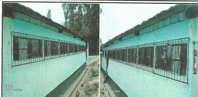
Foto 2: BALCONES: Mantenimiento de Balcones de Metal. -10 Balcones medidas 1.98 mts de ancho por 0.84 mts de altura
